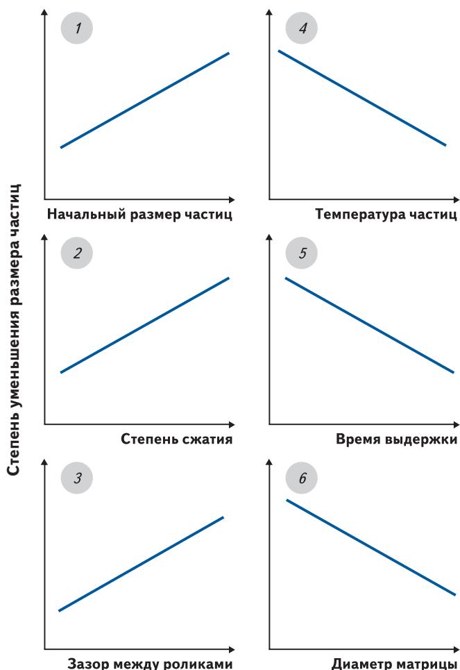
Рис. 2. Параметры, влияющие на степень уменьшения размера частиц: 1 — начальный размер частиц; 2 — степень сжатия; 3 — зазор между роликами; 4 — температура частиц; 5 — время выдержки; 6 — диаметр матрицы
