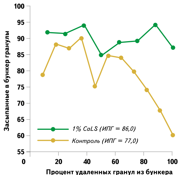
Рис. 3. Сегрегация россыпи в бункере с гранулами корма-финишера для индеек
