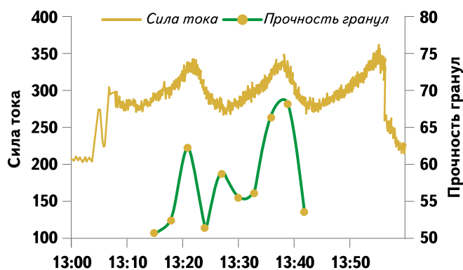
Рис. 1. Вариативность прочности гранул
