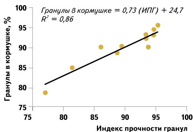
Рис. 2. Корреляция между ИПГ и гранулами в кормушке
